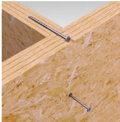
T-joint
